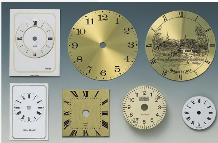
Zifferblätter, Barometer-, Thermometer-, Hygrometer-, Manometer-Skalen komplett gestanzt und verformt
